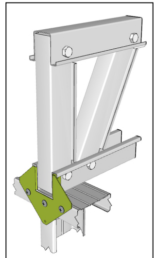
H1A Hold Down
